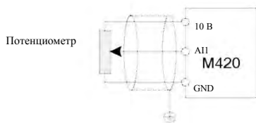
Рис. 3-10. Принципиальная схема для подключения входным клеммам аналогового сигнала.
