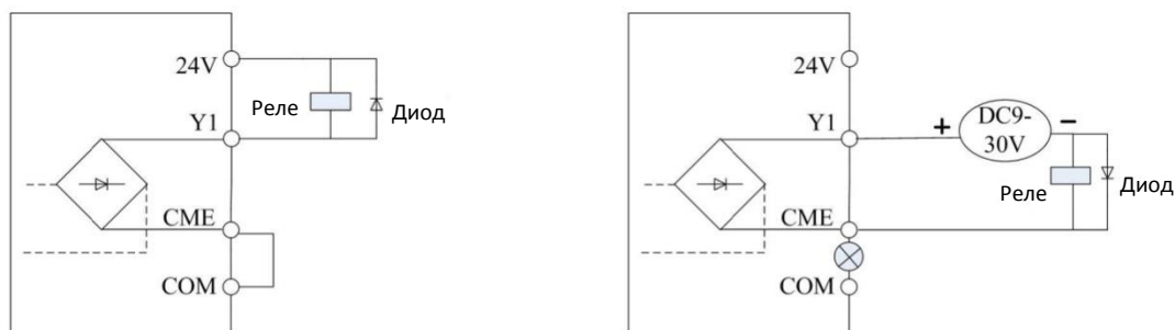
Внутренний источник питания
